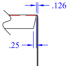
VIEW A-A SCALE: 3"=1'
