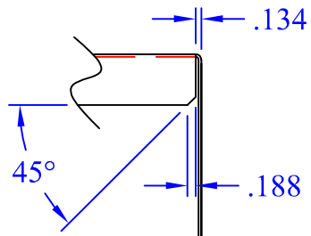
VIEW A-A SCALE: 3"=1'
