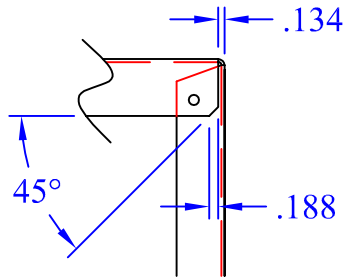
VIEW A-A SCALE: 3"=1'
