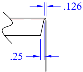
VIEW A-A SCALE: 3"=1'
