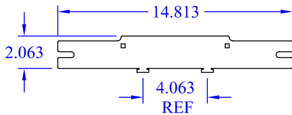
(4) WBT-2 IR
