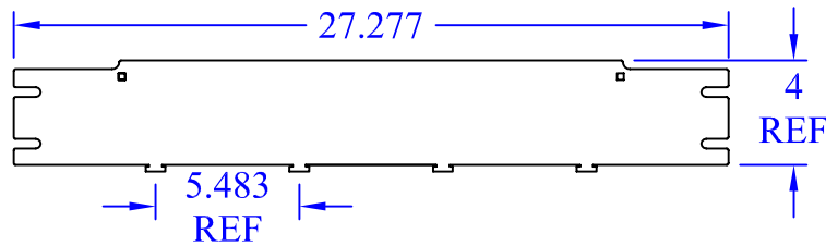
(1) WBT-90-6x8 OR
